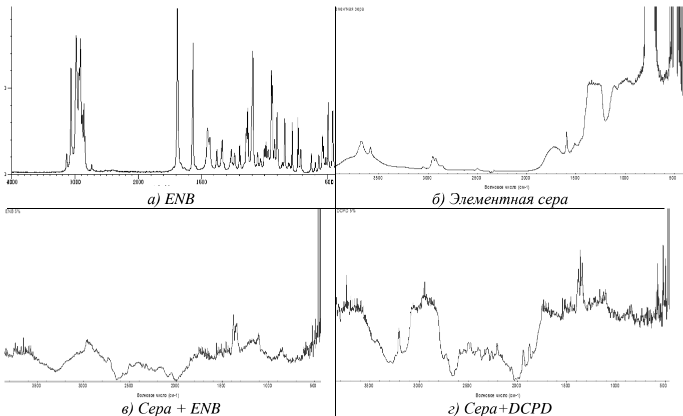
Рисунок 6 – ИК-спектры а) ENB; б) элементной серы; в) композиции серы с ENB г) композиции серы с DCPD
